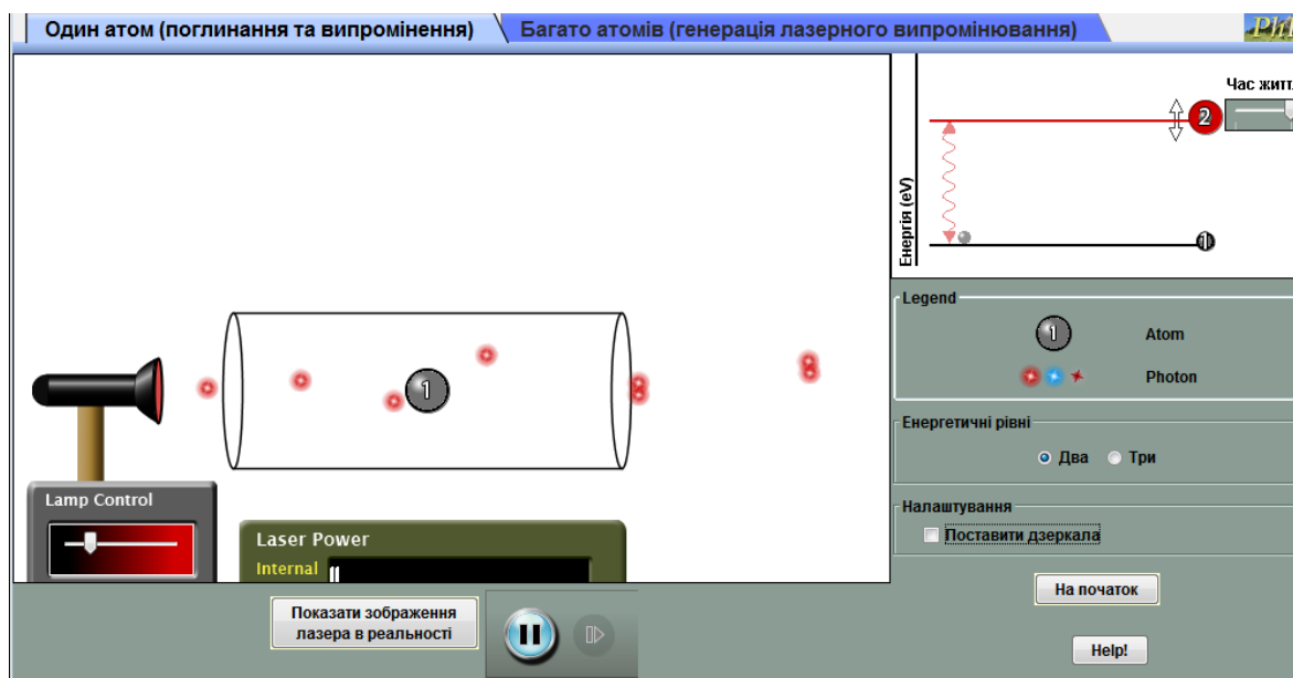
Рис. 1. Phet-симуляція «Лазери»
